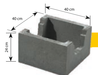
Pustak fundamentowy (z wpustem) symbol: D2 waga: ok. 30 kg
