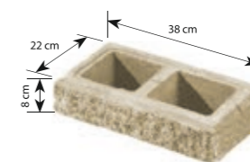
Pustak łupany symbol: A4 waga: ok. 8 kg
