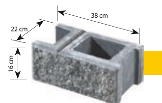
Pustak łupany (podmurówkowy) symbol: A1 waga: ok. 19,2 kg
