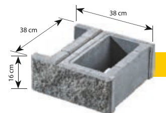
Pustak łupany (podmurówkowy) symbol: B1 waga: ok. 25,5 kg
