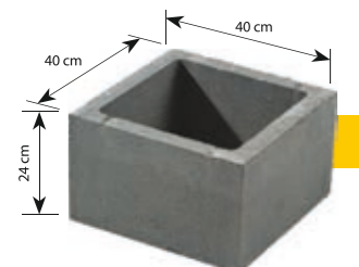
Pustak fundamentowy (pełny) symbol: D1 waga: ok. 33 kg
